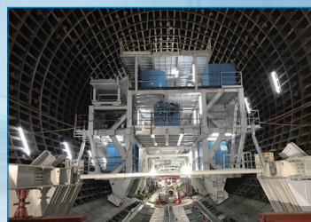
シールドマシン後続台車
